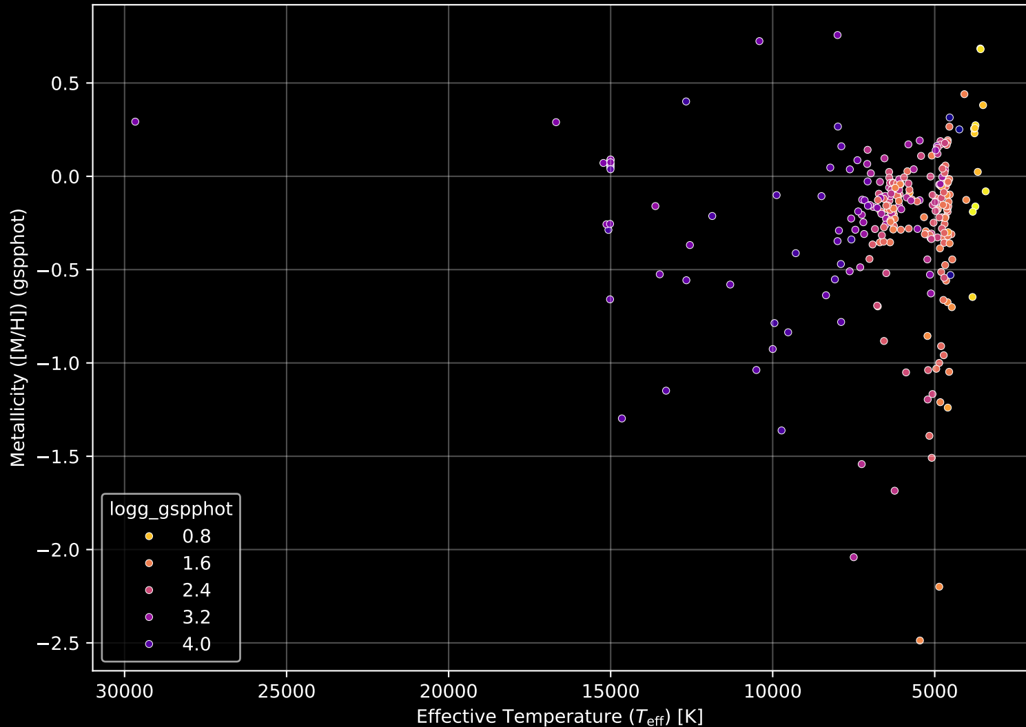
APOGEE DR17 Field: [139+00] Stellar Population Parameters (n= 271)
